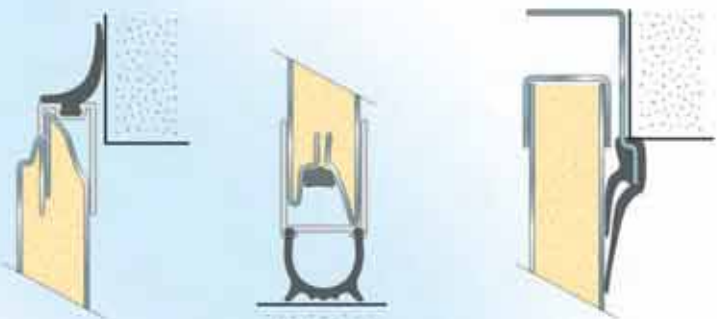
Topp, bunn og sidepakning
